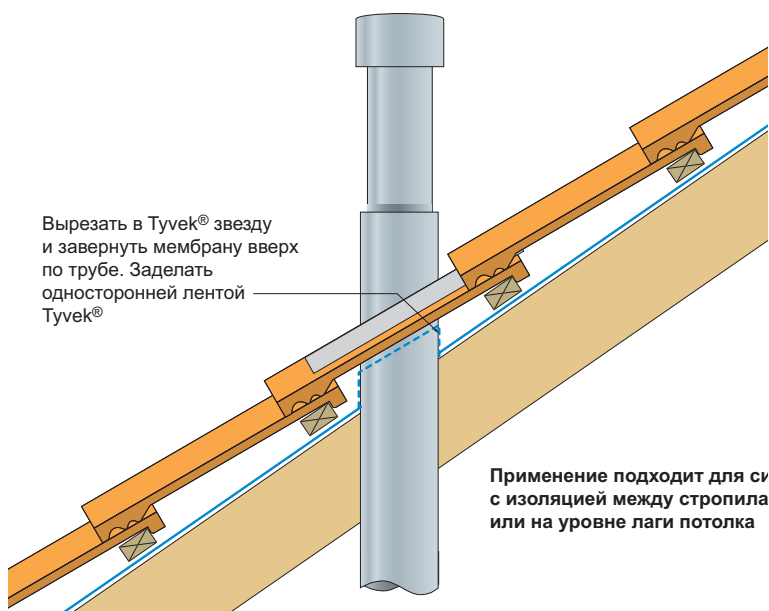
Рис. 45 - Вентиляционная труба
