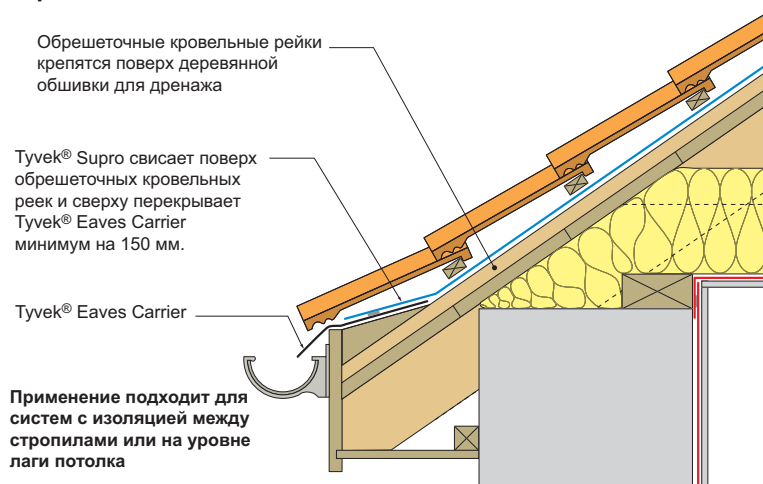
Рис.32 - Неподдерживаемая мембрана поверх деревянной обрешетки
